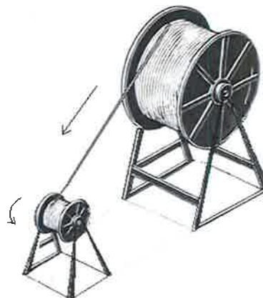
Rys. Prawidłowy sposób przewijania kabla z bębna na inny bęben
